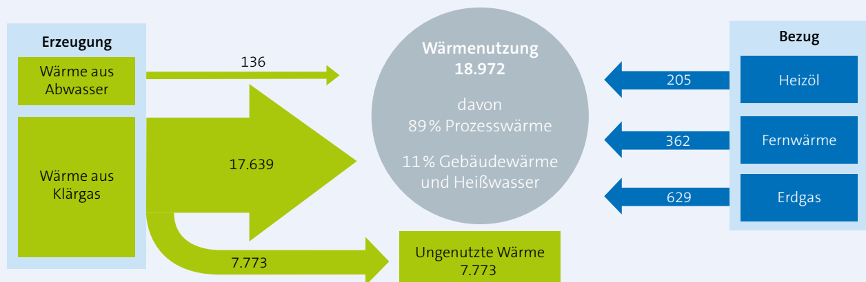
Wärmebilanz der hanseWasser 2021 in MWh
