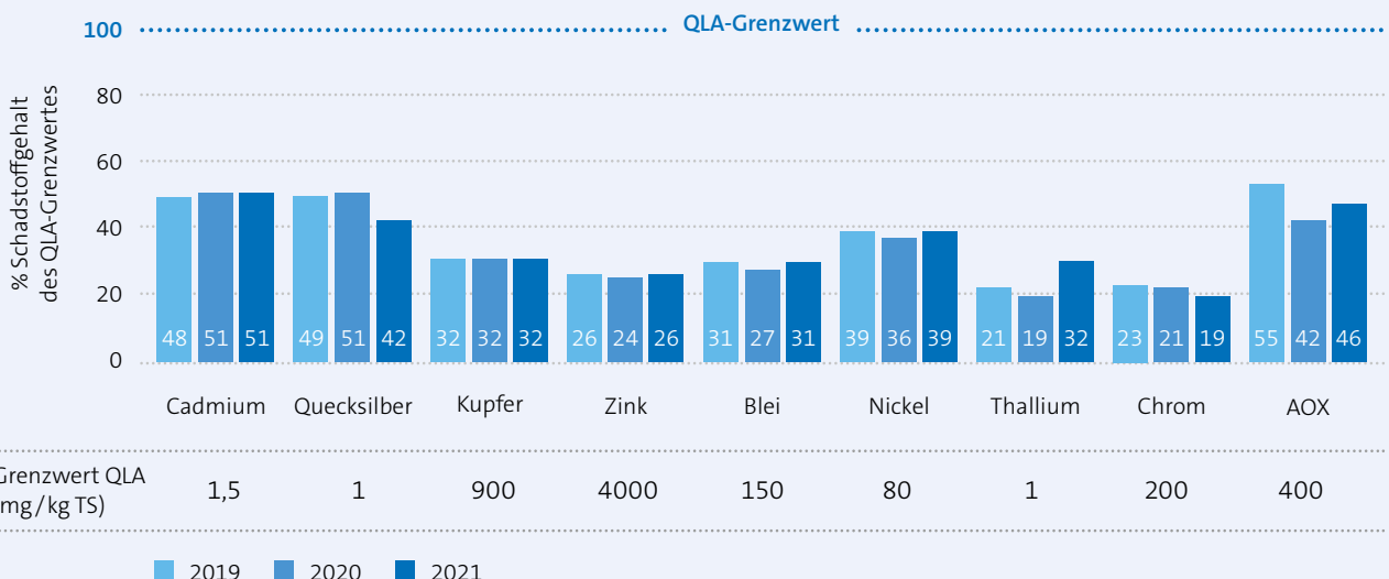
Schadstoffgehalte im Klärschlamm der Kläranlage Seehausen
