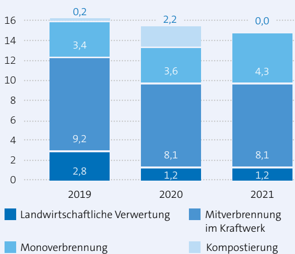
Verwertung der Klärschlämme in 1.000 t TR/a
