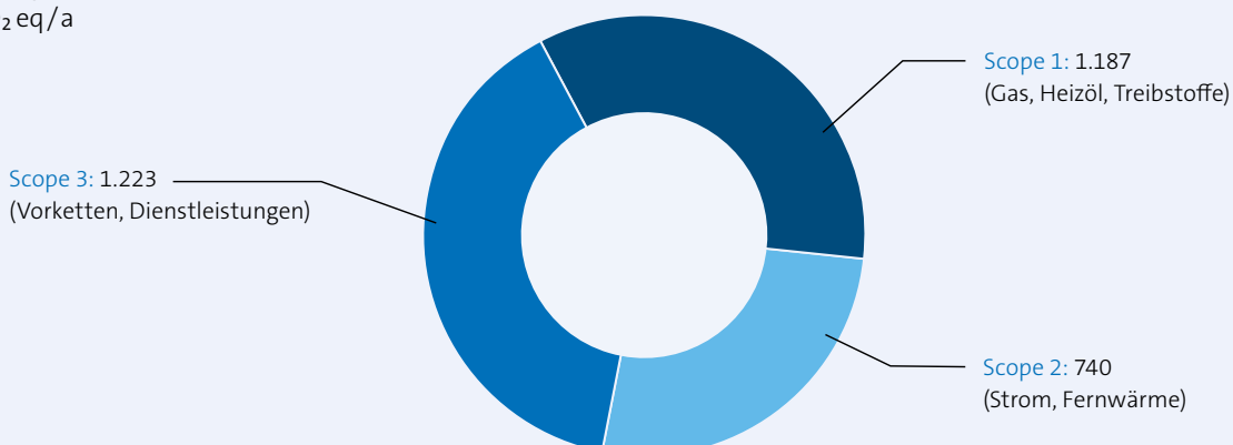
Einteilung der Emissionen bei hanseWasser 2021 in t CO 2 eq/a
